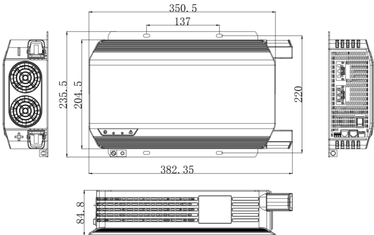
Figure 2-5 Dimension du convertisseur Série NH
