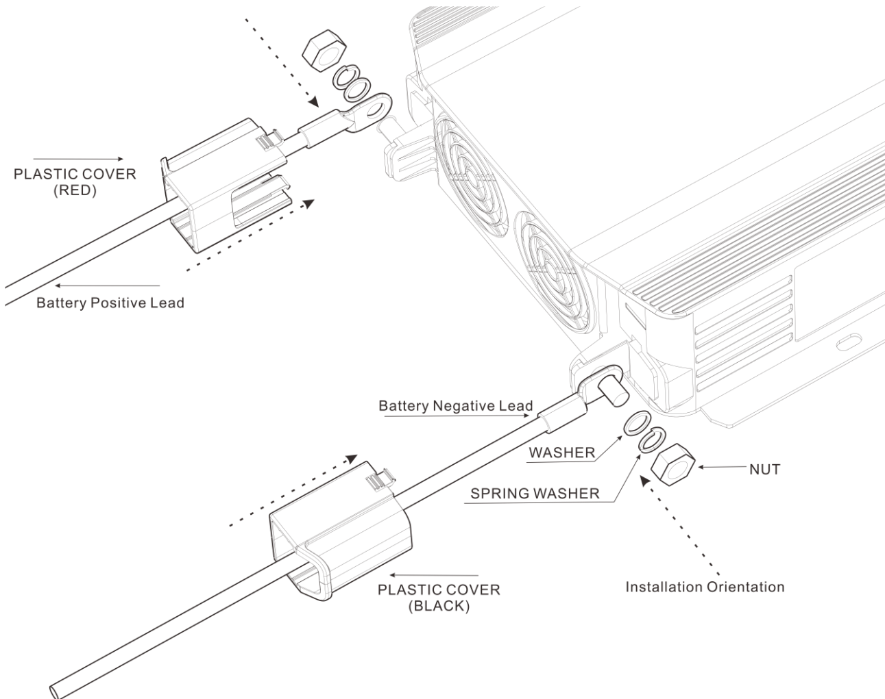
Abbildung 3-2 DC-Kabelanschlußdiagramm für NH
