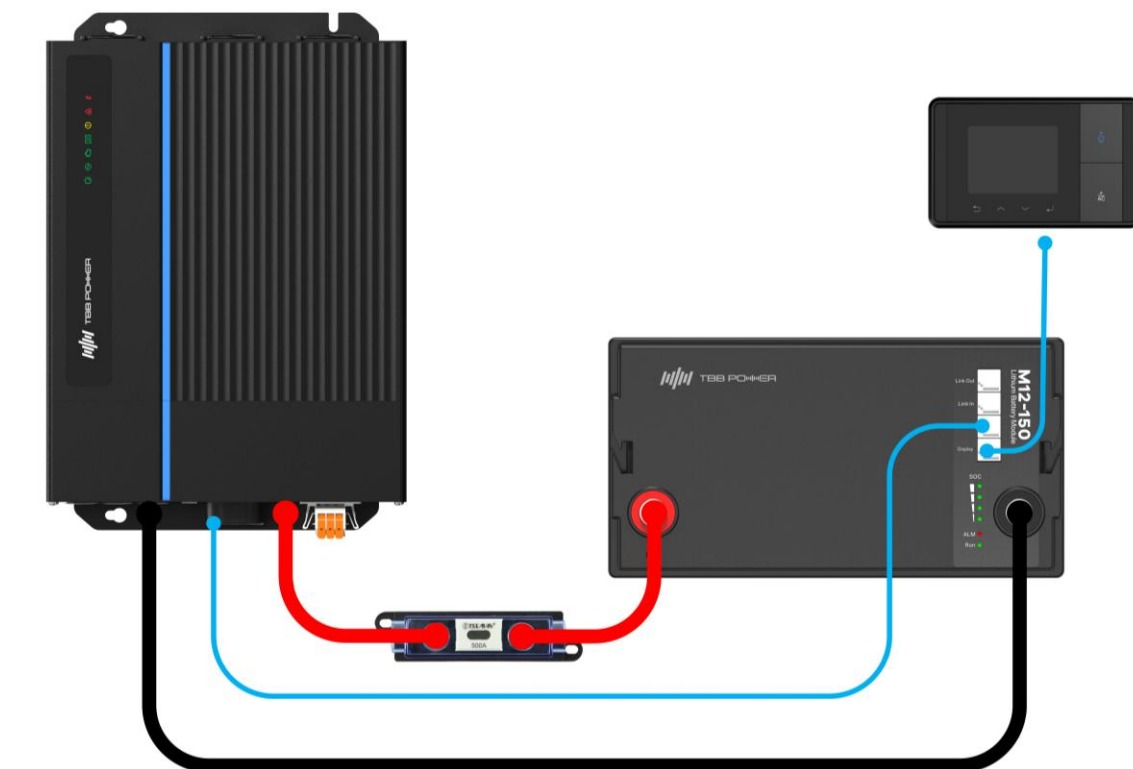
Bild 2-4 Typischer Verdrahtungsplan
