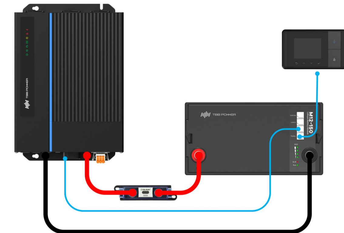
Figure 2-4 Schéma de câblage type
