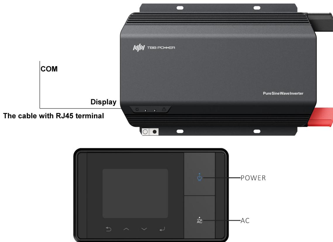
Abbildung 2-6: Anschlussdiagramm zwischen NH-Wechselrichter und VS28-LS-Display
