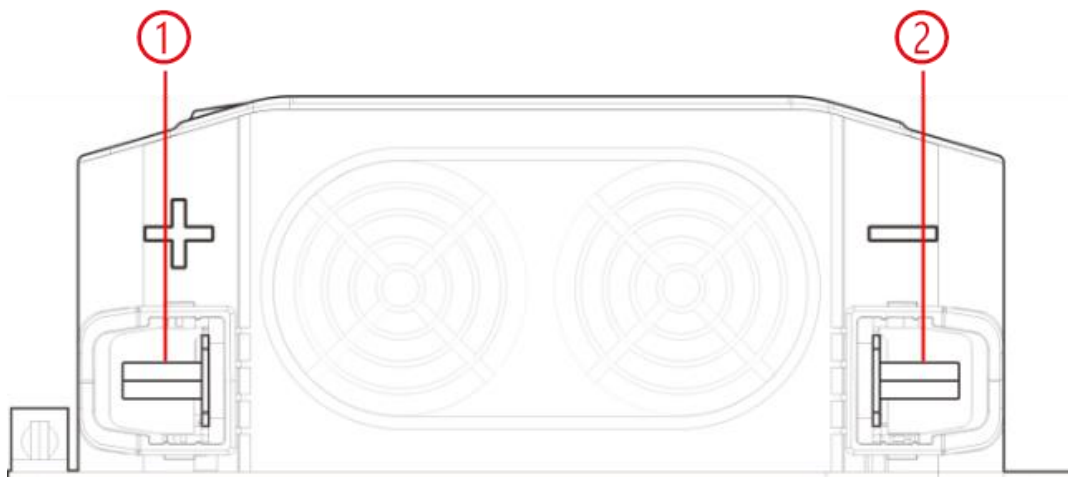
Abbildung 2-2: Anschlüsse auf der DC-Seite
