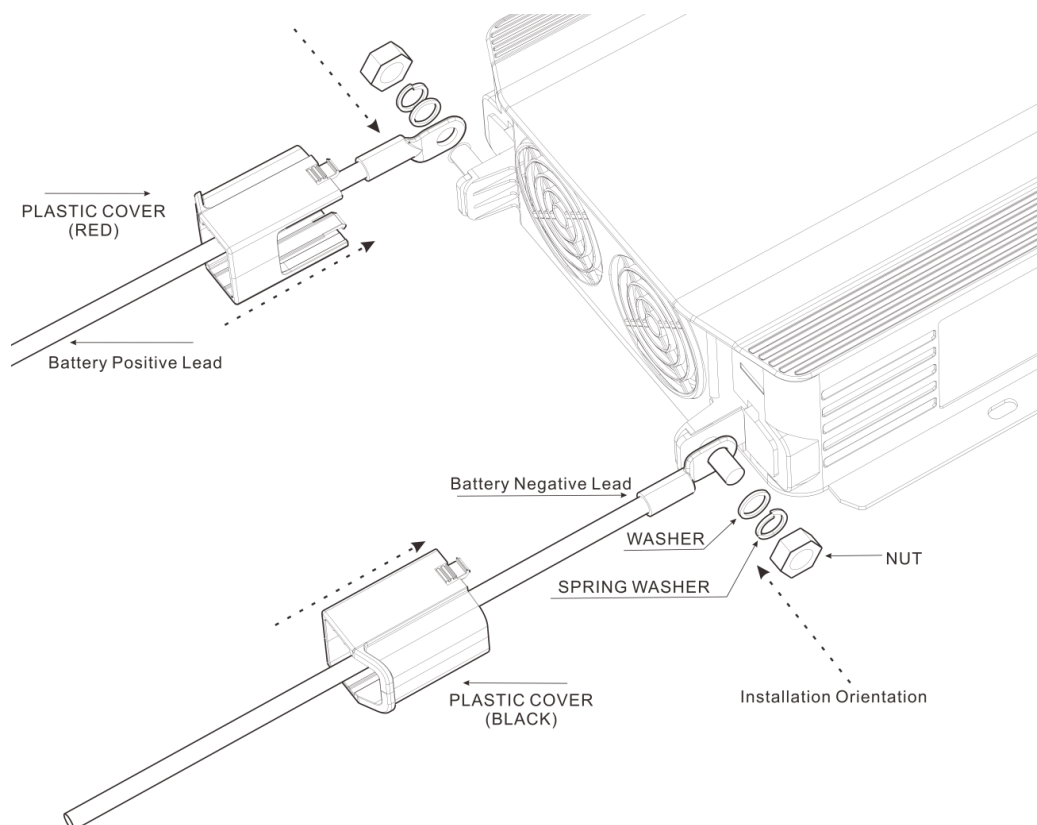
Figure 3-2 Schéma de connexion des câbles CC pour le convertisseur Série NH
