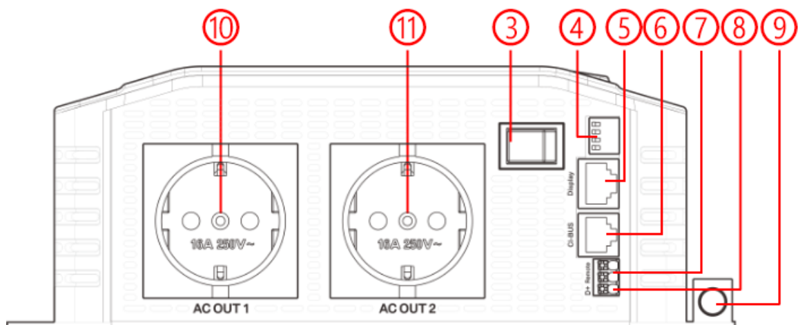
Abbildung 2-3: AC-Strom- und Signalanschlüsse für Modelle ohne Bypass-Funktion
